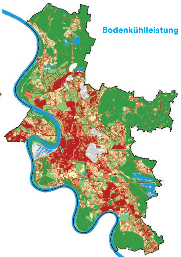
Bodenfunktionsbewertung
