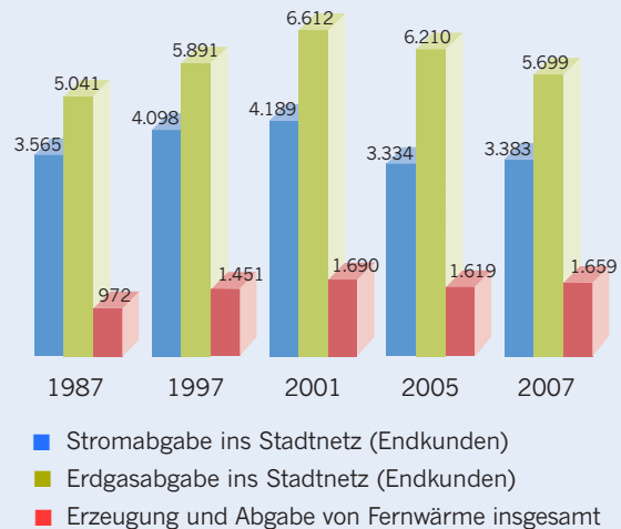
Strom-, Erdgas- und Fernwärmeabgabe Gigawattstunden (GWh)
