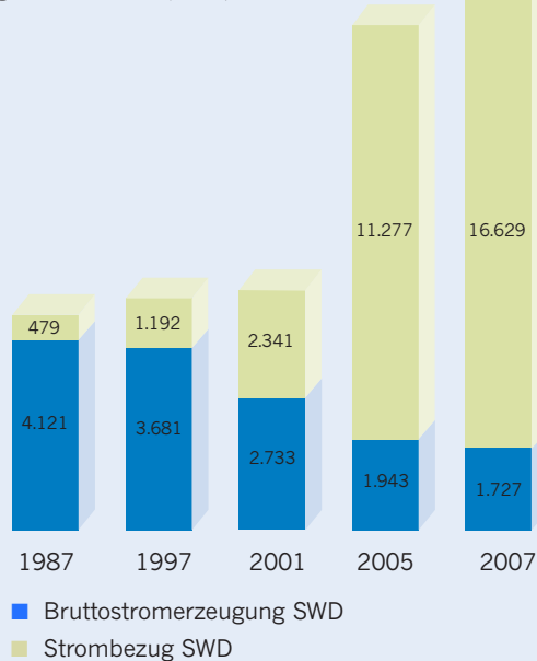
Stromerzeugung und Strombezug Gigawattstunden (GWh)
