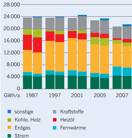
Vergleich des Endenergieverbrauchs 1987-2007 1. Säule Standard, 2. Säule ecospeed
