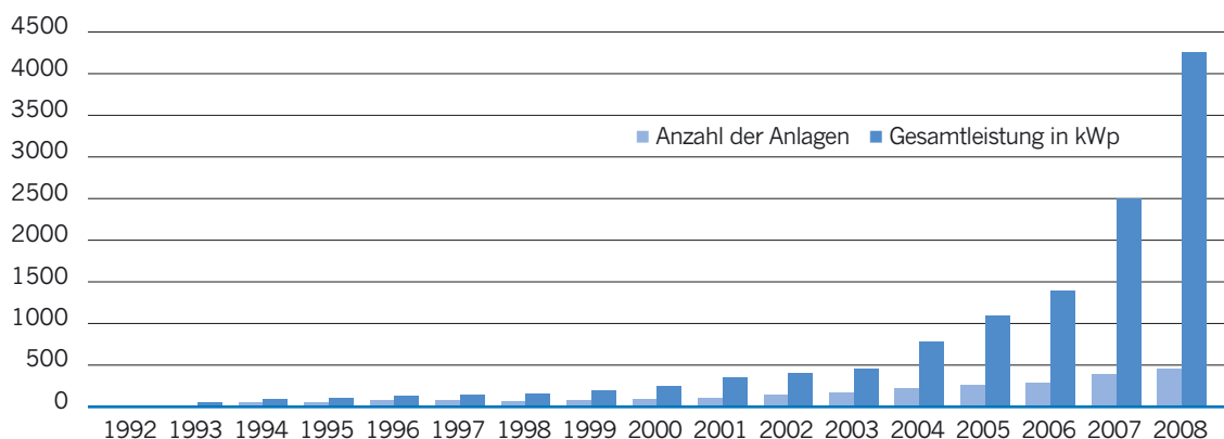
Anzahl und Gesamtkapazität der installierten Fotovoltaikanlagen in Düsseldorf
