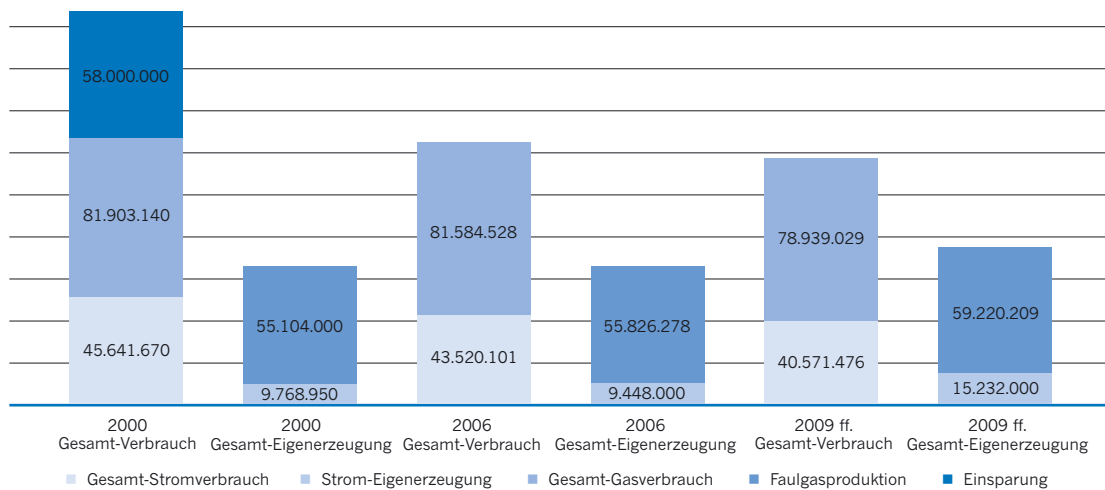
Vergleich Strom- und Gasverbrauch/Eigenerzeugung (Ausblick) in Kilowattstunden
