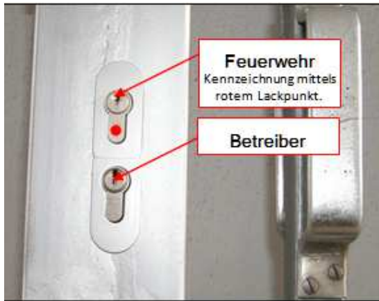
Beispiel Doppelschließung (Ausführung Zylinder nebeneinander auch möglich)
