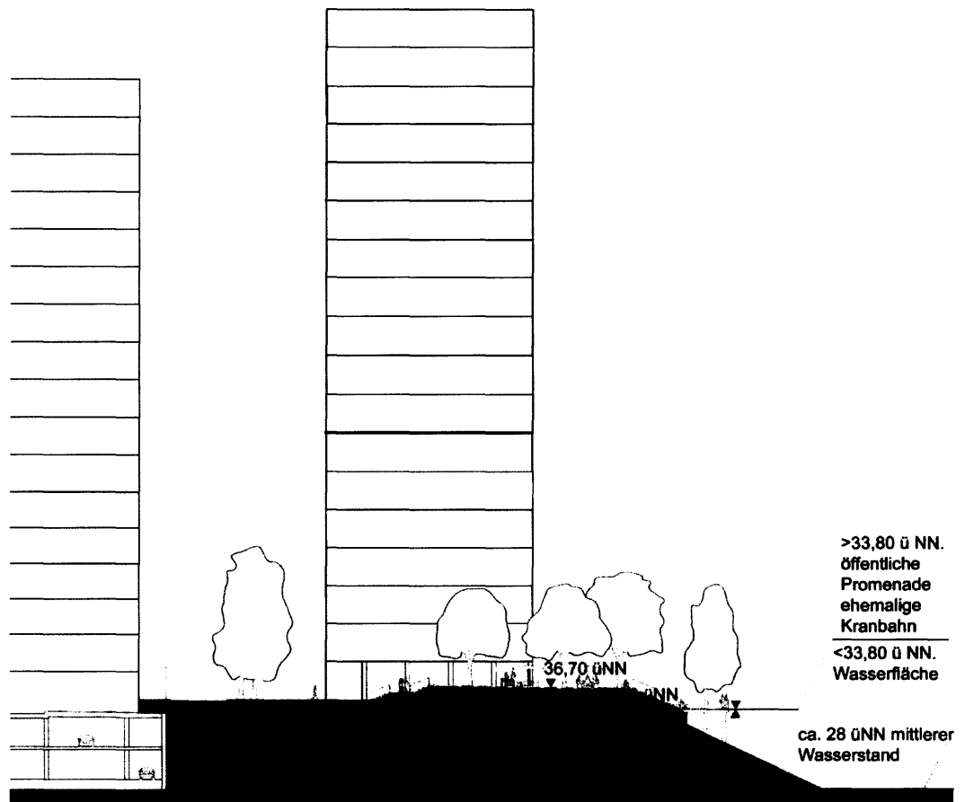
Abbildung 2: Schnitt mit der Lage der festgesetzten Fußgängerpromenade (ehemalige Kranbahn)
