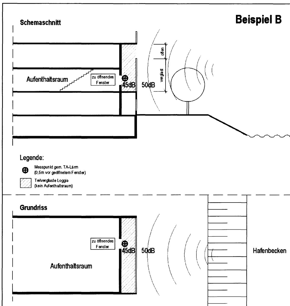
Abbildung 4: Beispiel B für die Anordnung einer teilverglasten Loggia (schematische Darstellung)
