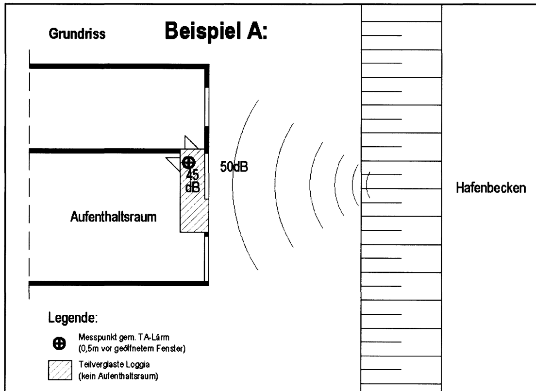
Abbildung 3: Beispiel A für die Anordnung einer teilverglasten Loggia (schematische Darstellung)
